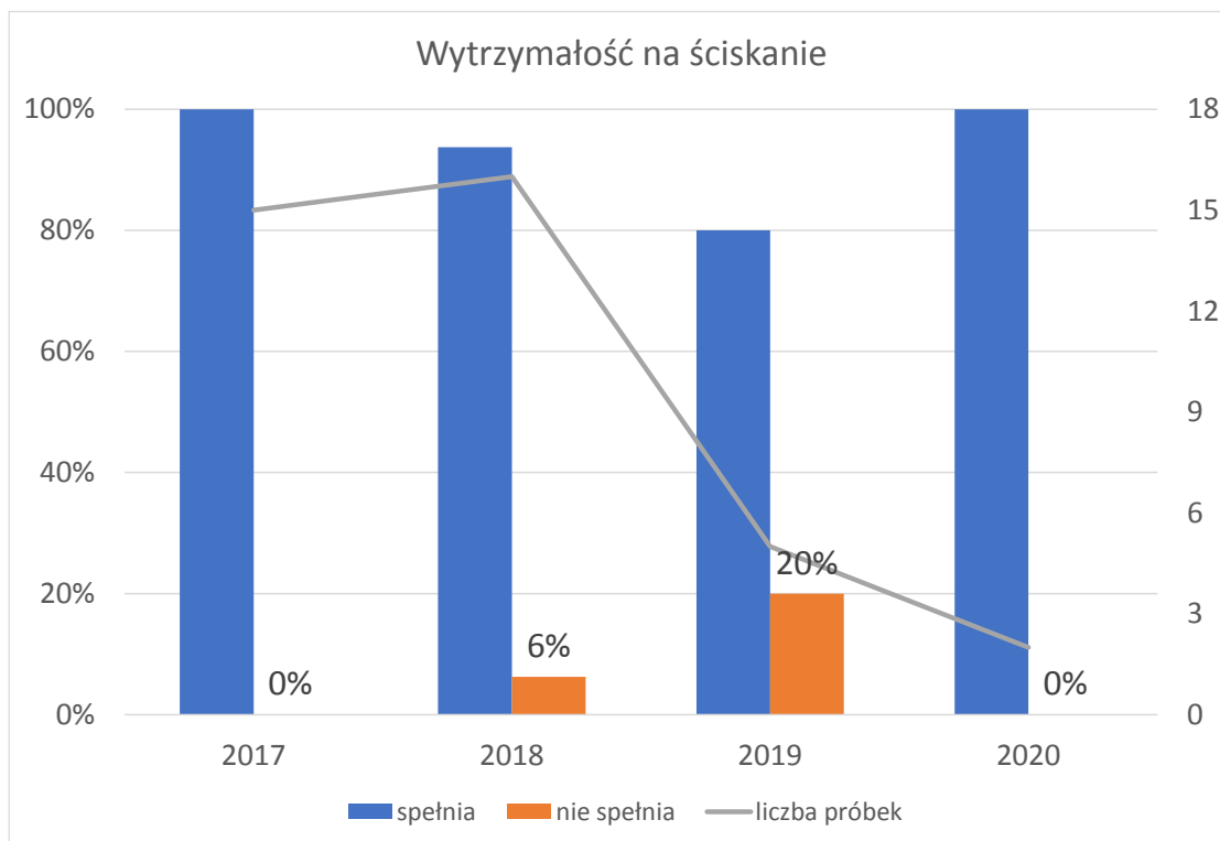
Rysunek 38 Spełnienie wymagania dotyczącego wytrzymałości na ściskanie przez elementy murowe w latach 2017-2020
