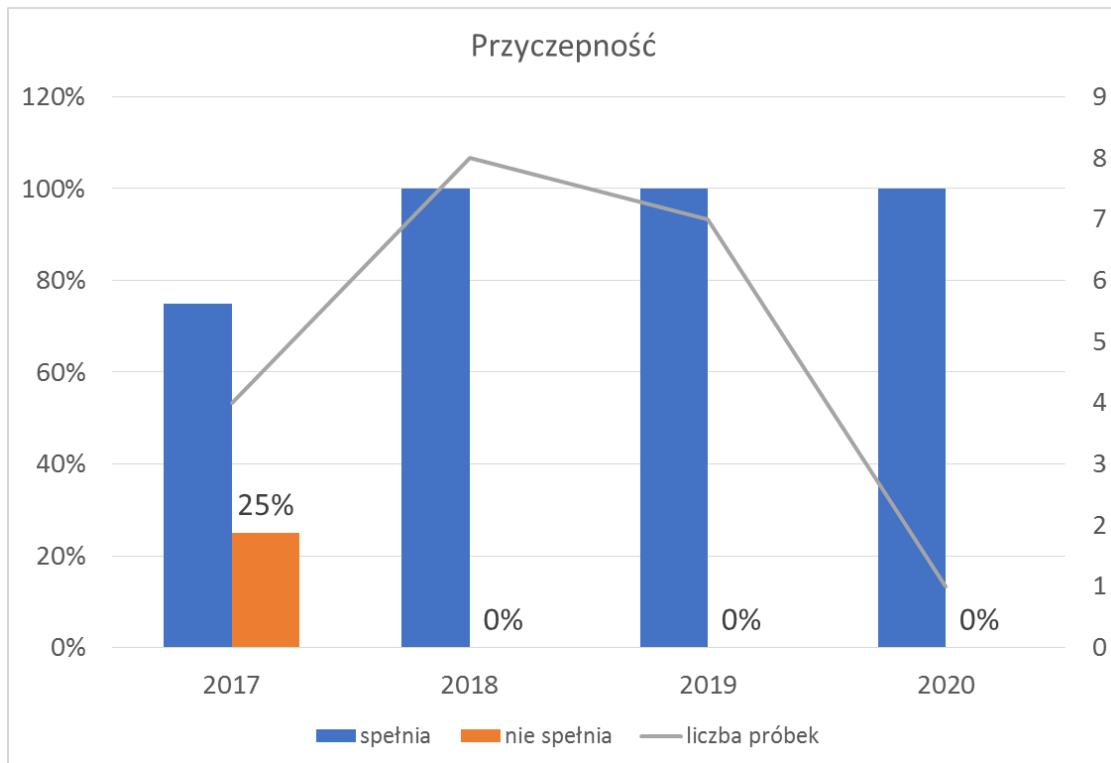
Rysunek 42 Spełnienie wymagania dotyczącego przyczepności przez zaprawy tynkarskie i murarsko-tynkarskie w latach 2017-2020
