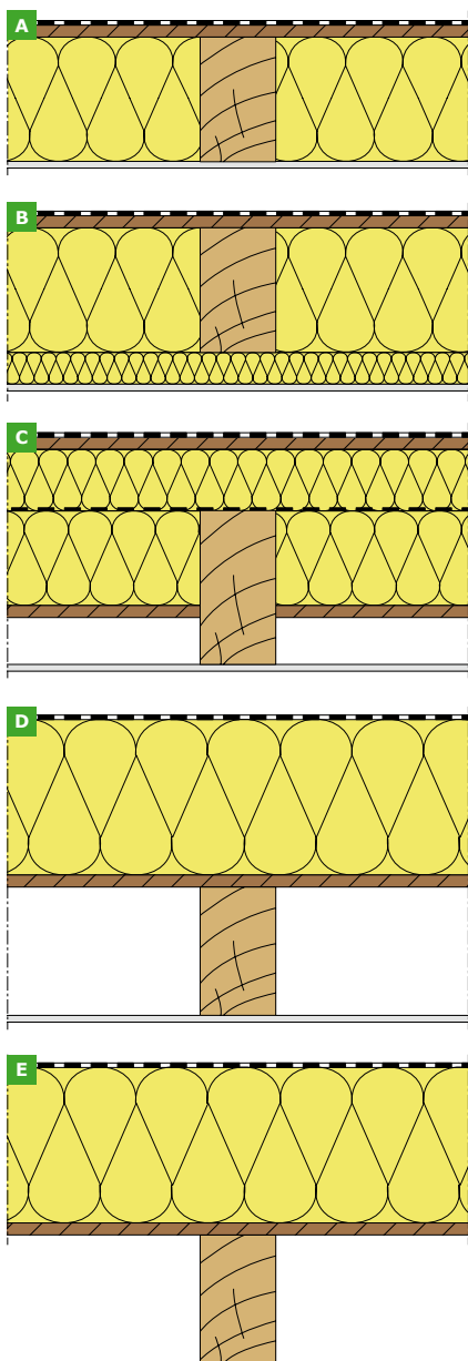
RYŚ. 22. Przykłady stropodachów pełnych opartych na drewnianych krokwiach (opisy w tekście); rys.: [2–3]
