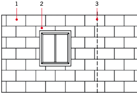
RYS. 2. Układ płyt styropianowych na powierzchni ściany
