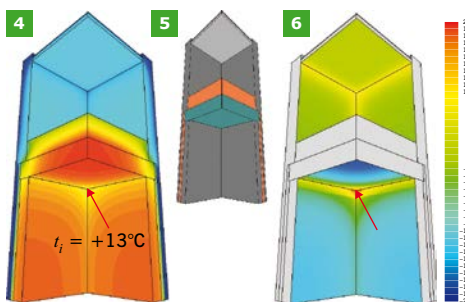
RYS. 4–6. Ocieplenie stropu j.w., lecz grubości 20 cm (docieplenie nową warstwą grubości 15 cm): pola rozkładu temperatury (4), model przegrody (5), pola rozkładu strumienia ciepła (6); rys.: autor
