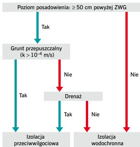
RYS. 2. Procedura doboru rodzaju uszczelnienia na podstawie warunków gruntowo-wodnych; rys.: autor
