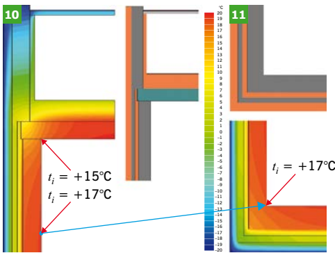
RYS. 10–11. Przekrój dla modelu z RYS. 7–9: pionowy przekrój przez stropodach (10), poziomy przez narożnik wypukły ścian (11); rys.: autor
