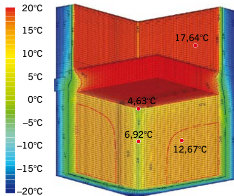
RYS. 4. Naroże dolne – ściany powyżej stropu ocieplone; temperatura t_{ND1} w narożu płaskim 2D t_{ND1} = 6,92^{\circ}\text{C} , temperatura w narożu 3D t_{ND2} = 4,63^{\circ}\text{C} ; rys.: autorzy
