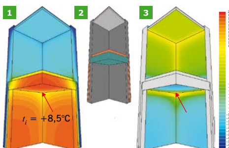
RYS. 1–3. Typowe ocieplenie stropodachów w pierwszych rozwiązaniach systemu W-70 (warstwa izolacji grubości 5 cm): pola rozkładu temperatury (1), model przegrody (2), pola rozkładu strumienia ciepła (3); rys.: autor
